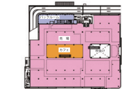
2階平面図
